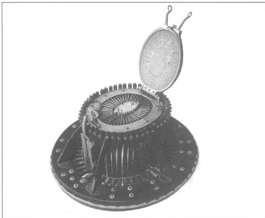
Fig. 8 - Conformador da marca Allié-Maillard.
